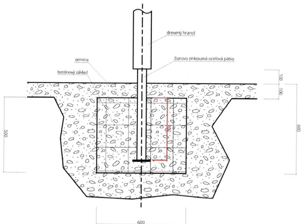
Detail ukotvenia
