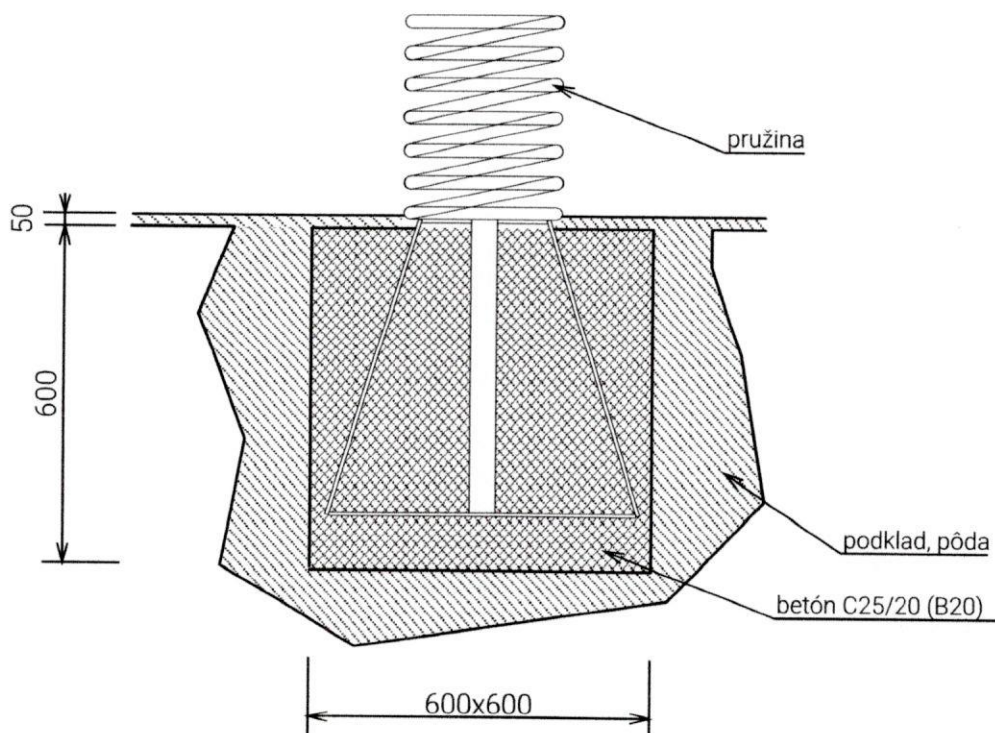
Detail ukotvenia
